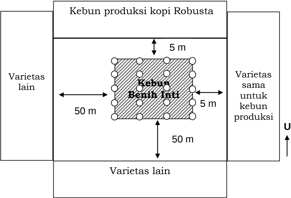
Gambar 1. Tata Tanam/Desain Kebun Induk Kopi Arabika Lahan Datar
